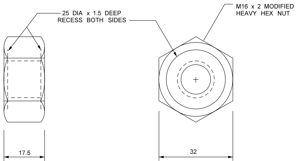
DETAILS 1:1
