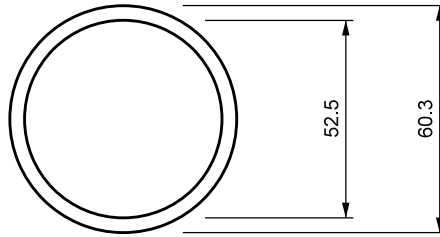
PLAN 1:2
